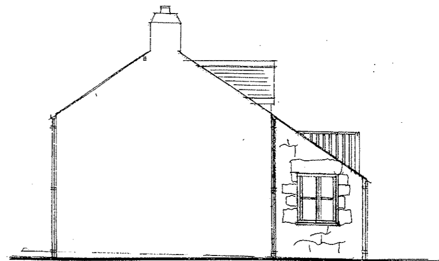
N.W. ELEVATION
