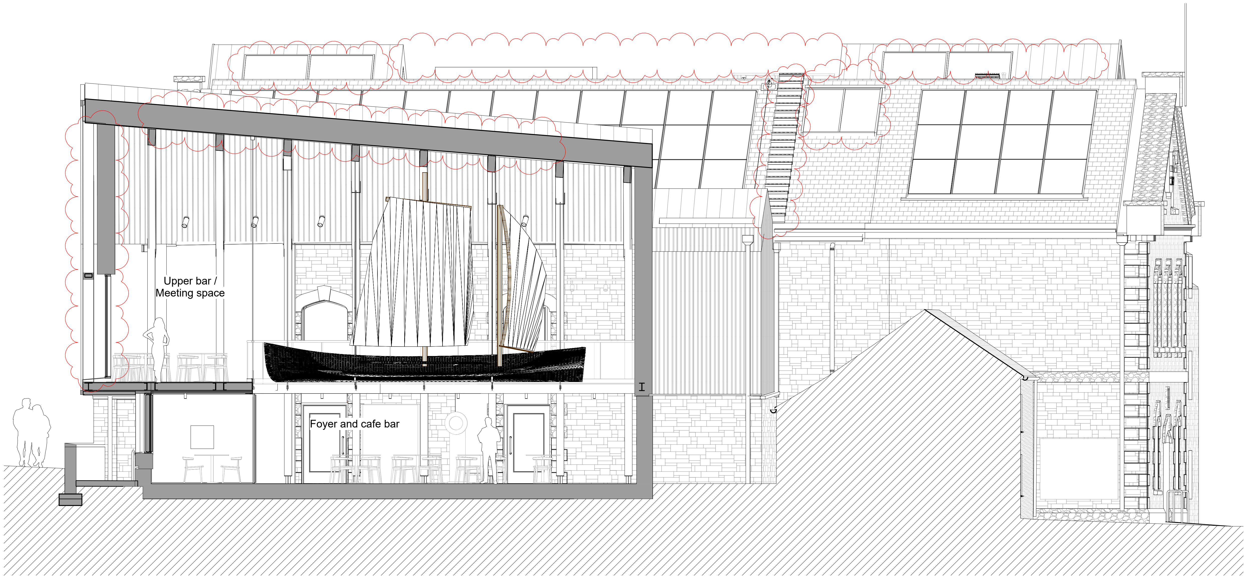
1 Section B-B 1 : 50
