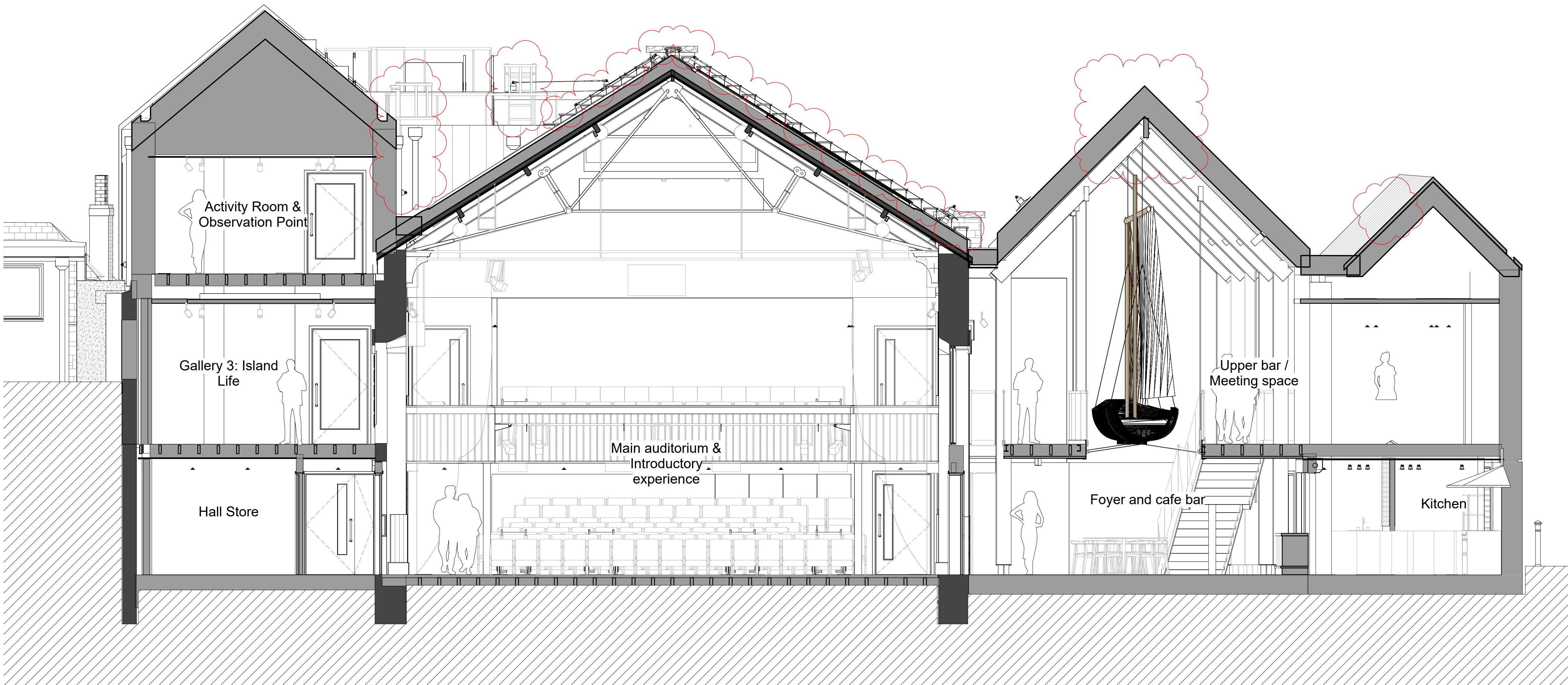
1 Section C-C 1 : 50
