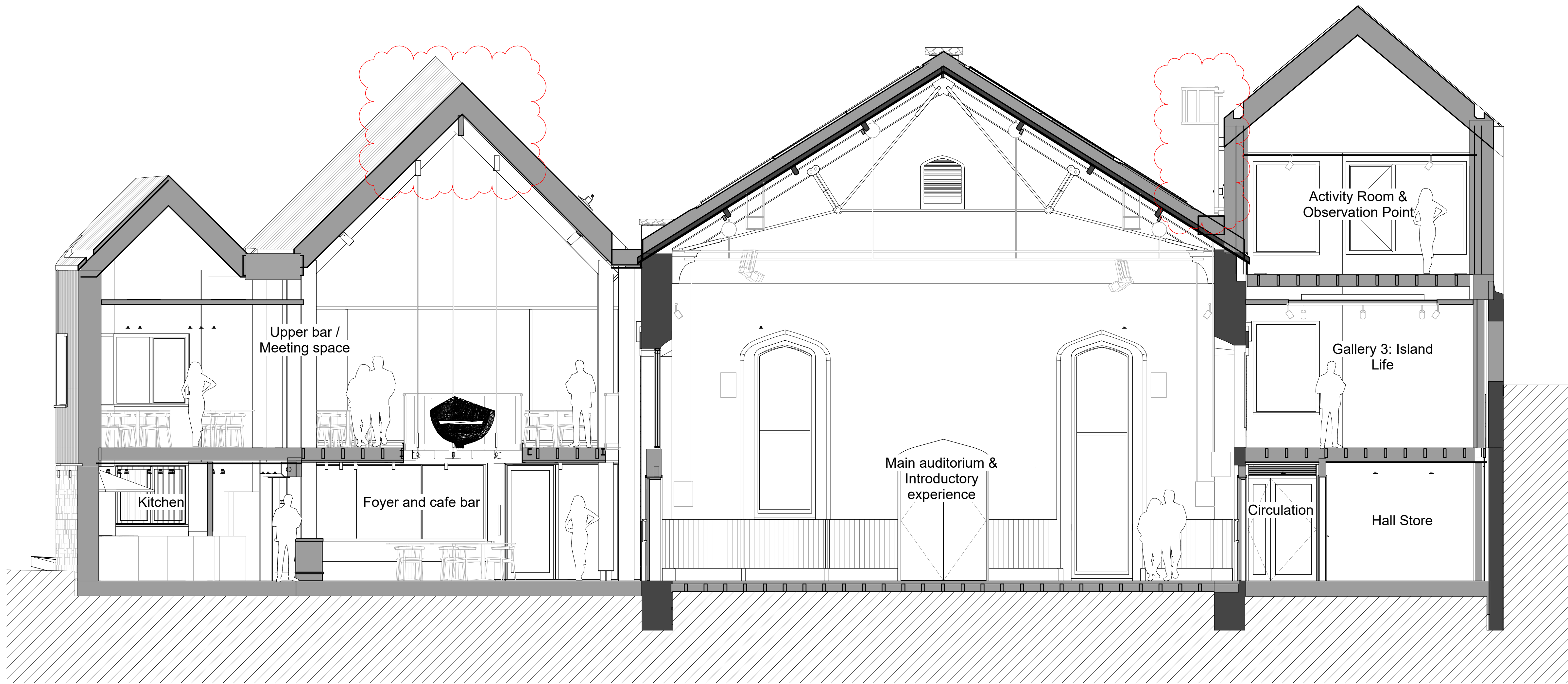
1 Section D-D 1 : 50
