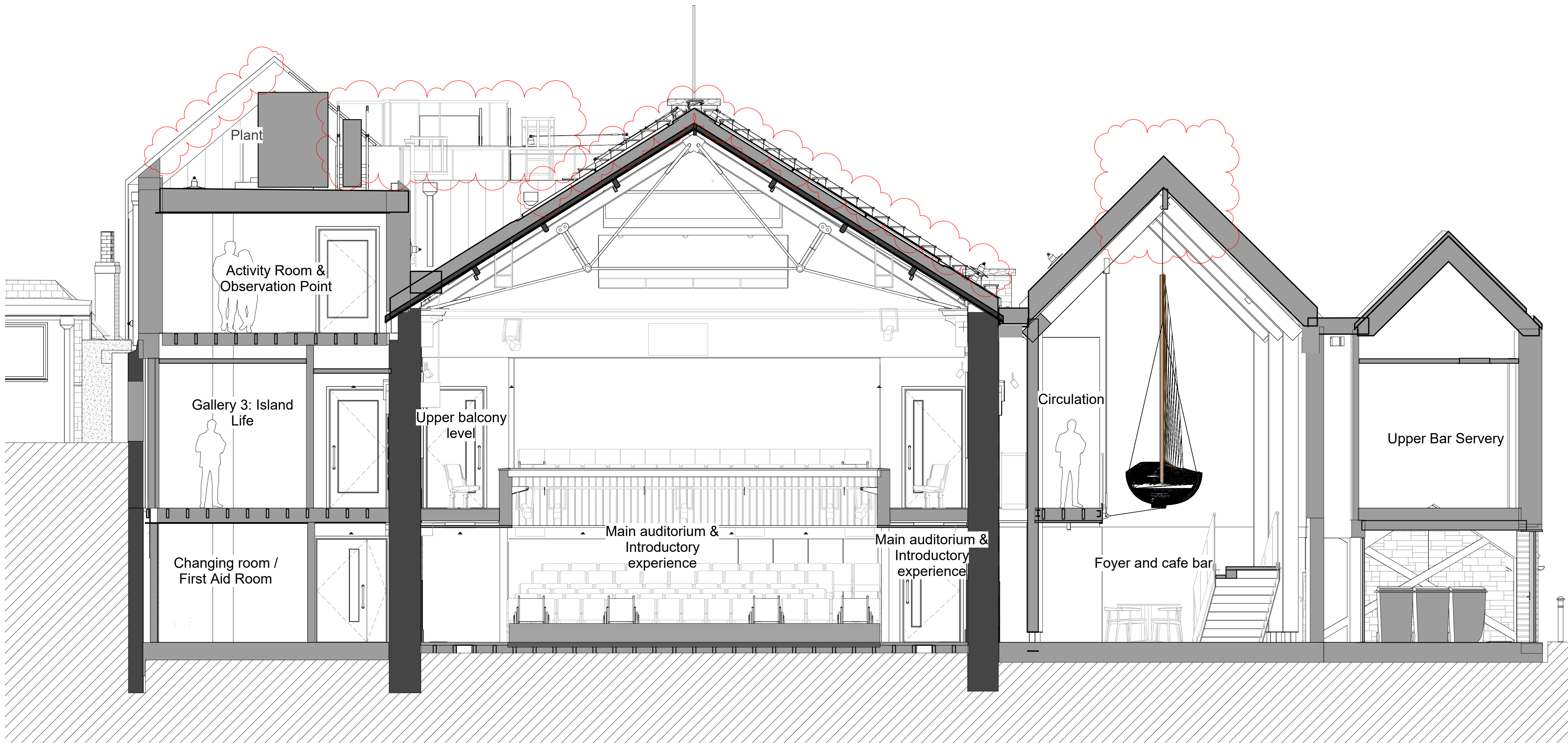
1 Section G-G 1 : 50
