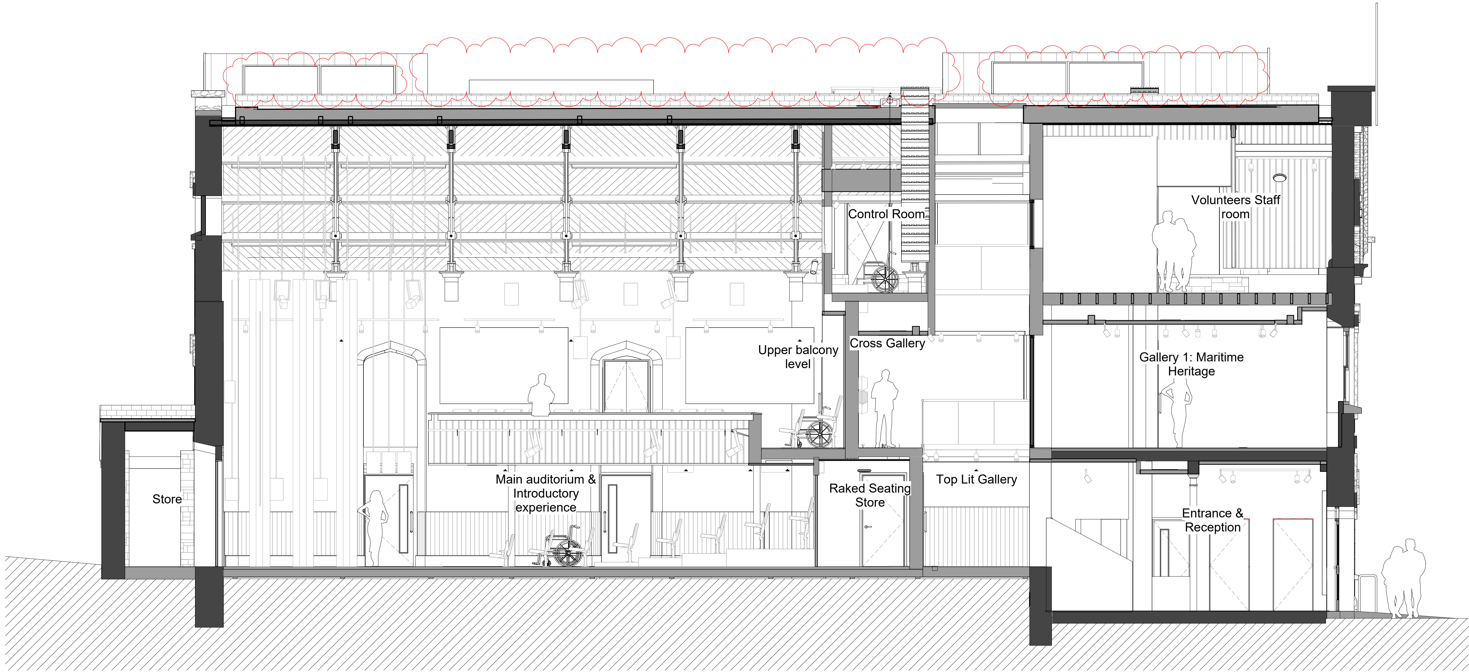
1 Section A-A 1 : 50
