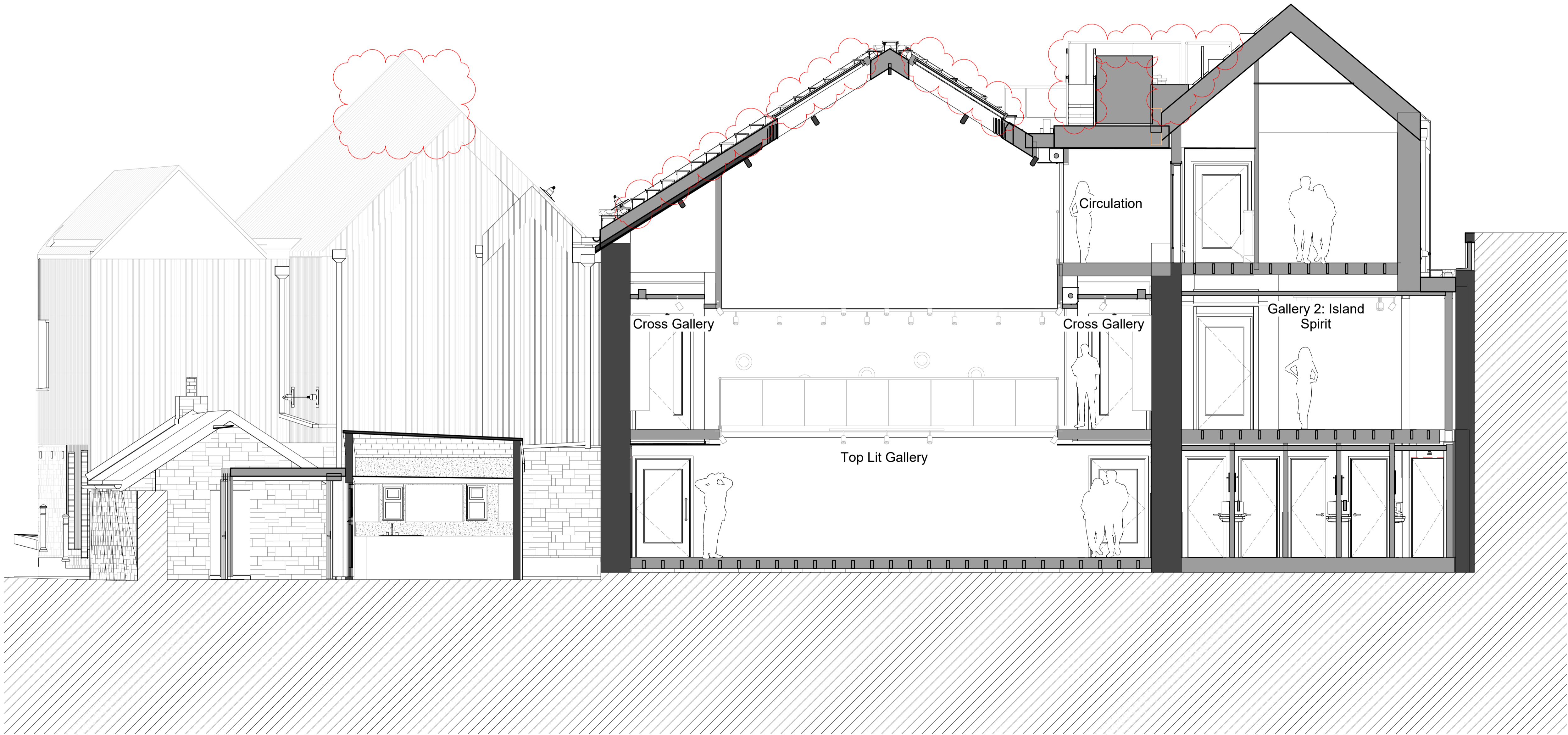
1 Section E-E 1 : 50
