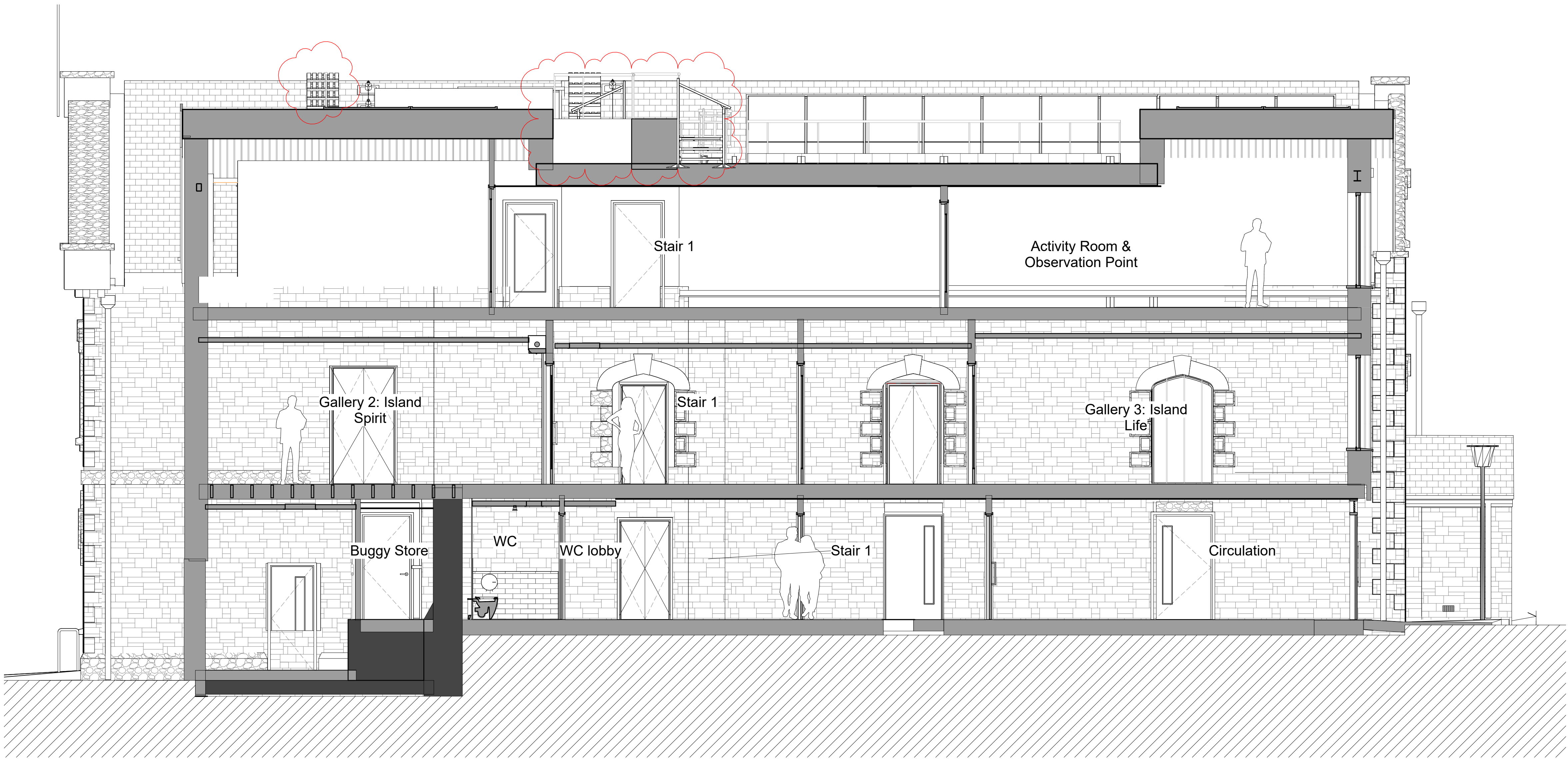
1 Section F-F 1 : 50
